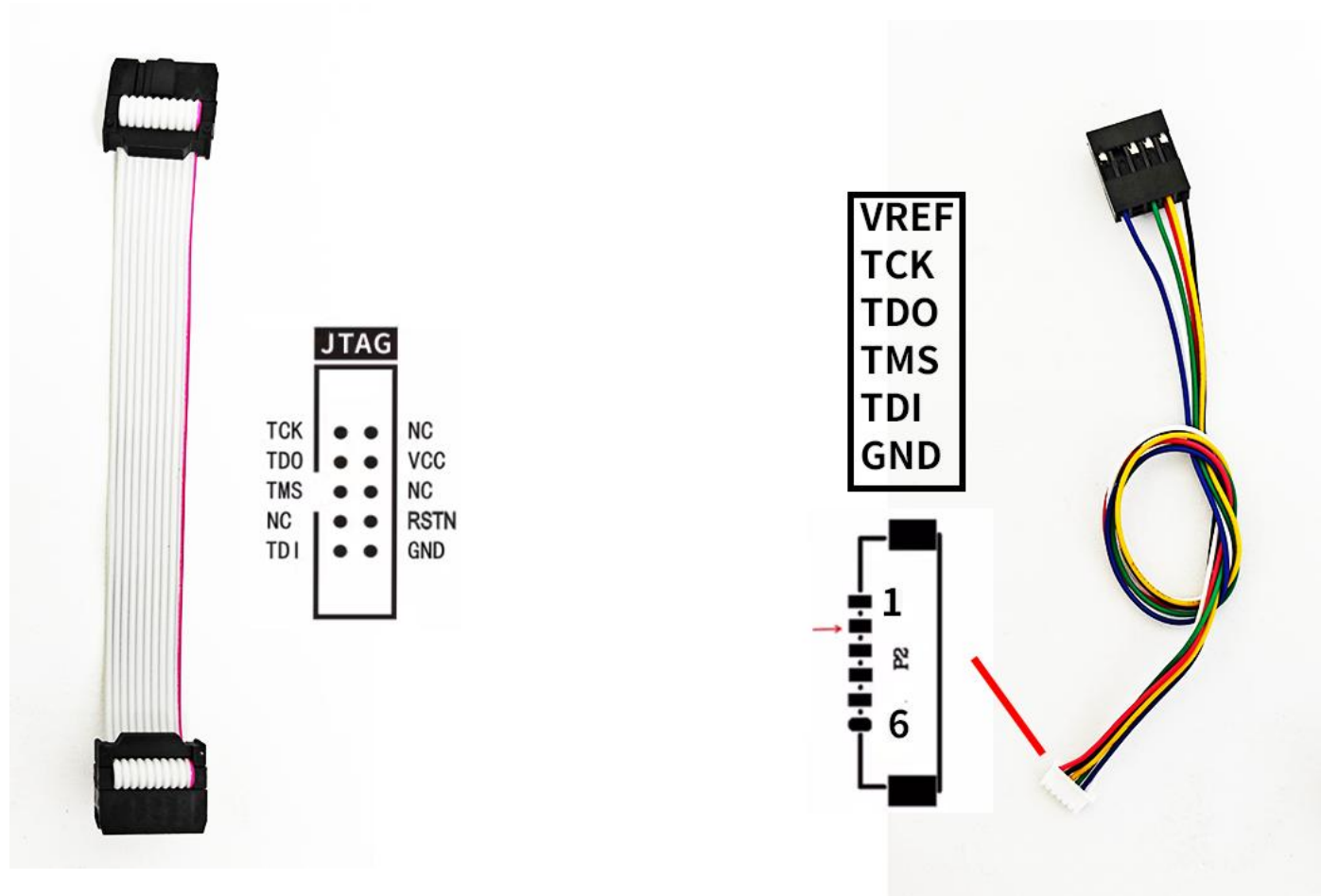
▲ 传统JTAG口
